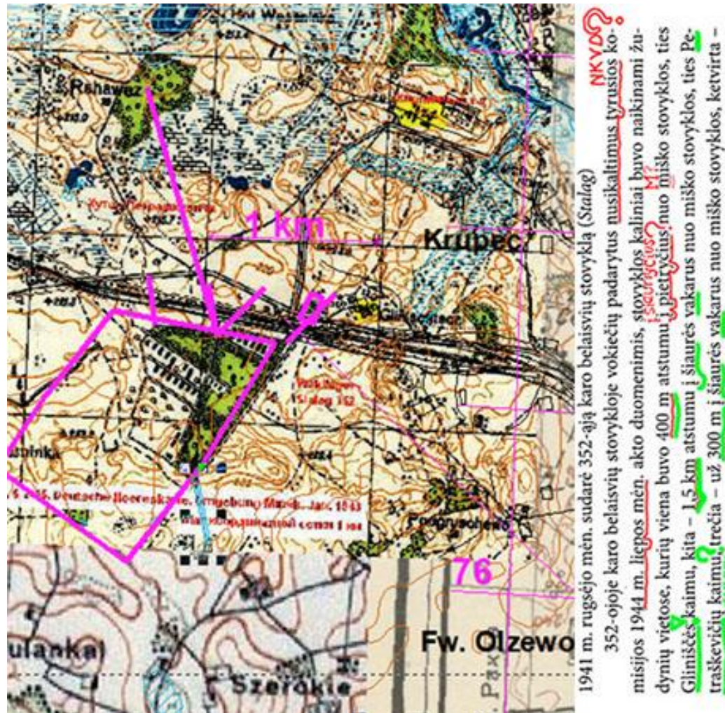
28 pav. : ant lenkiško 1930-ųjų metų žemėlapiu uždėto 1940-ųjų metų vokiškojo reljefo situacija ir apie žudynių vietas A. Bubnio nurodytų atstumų ir krypčių violetinės
